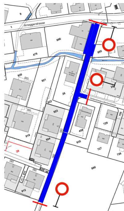
Übersicht Deckbelagseinbau
